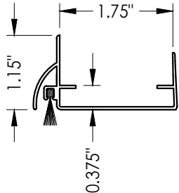
45 DOOR SWEEP
